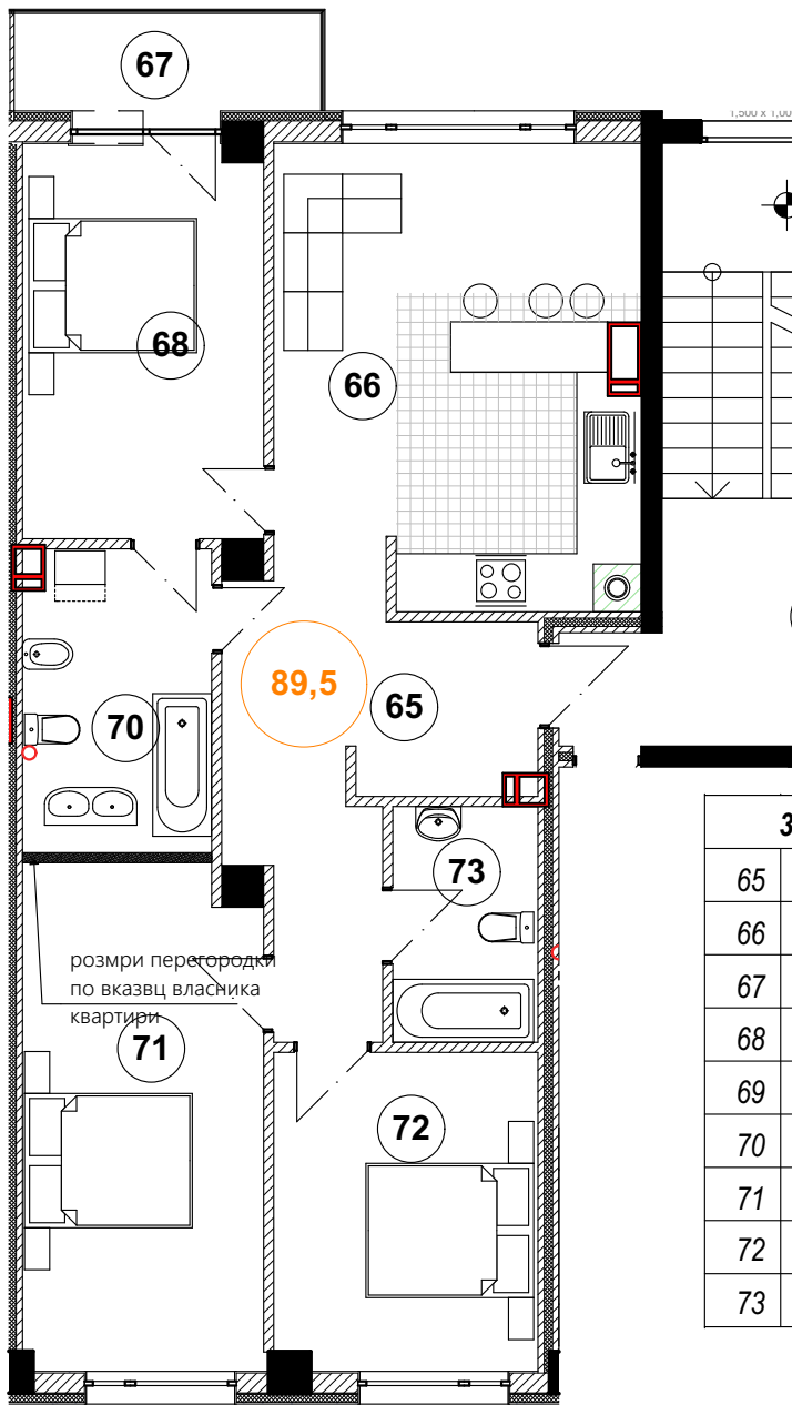
Схема секції
